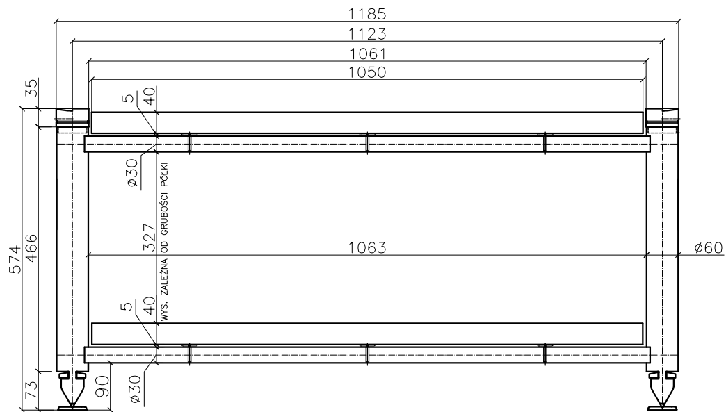
PRZEKRÓJ B-B
